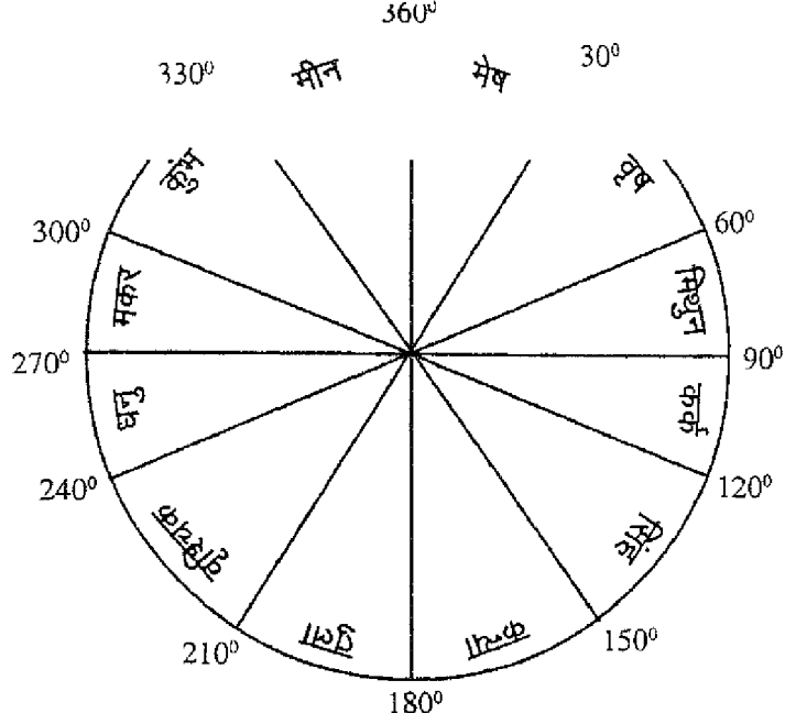
चित्र-1 पृथ्वी के परिपथ में राशियों का विभाजन
